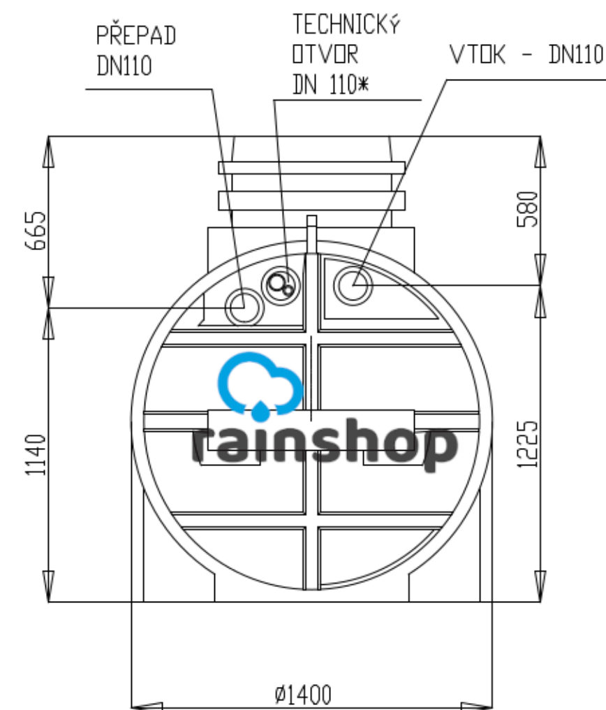
BOČNÍ POHLED 2
